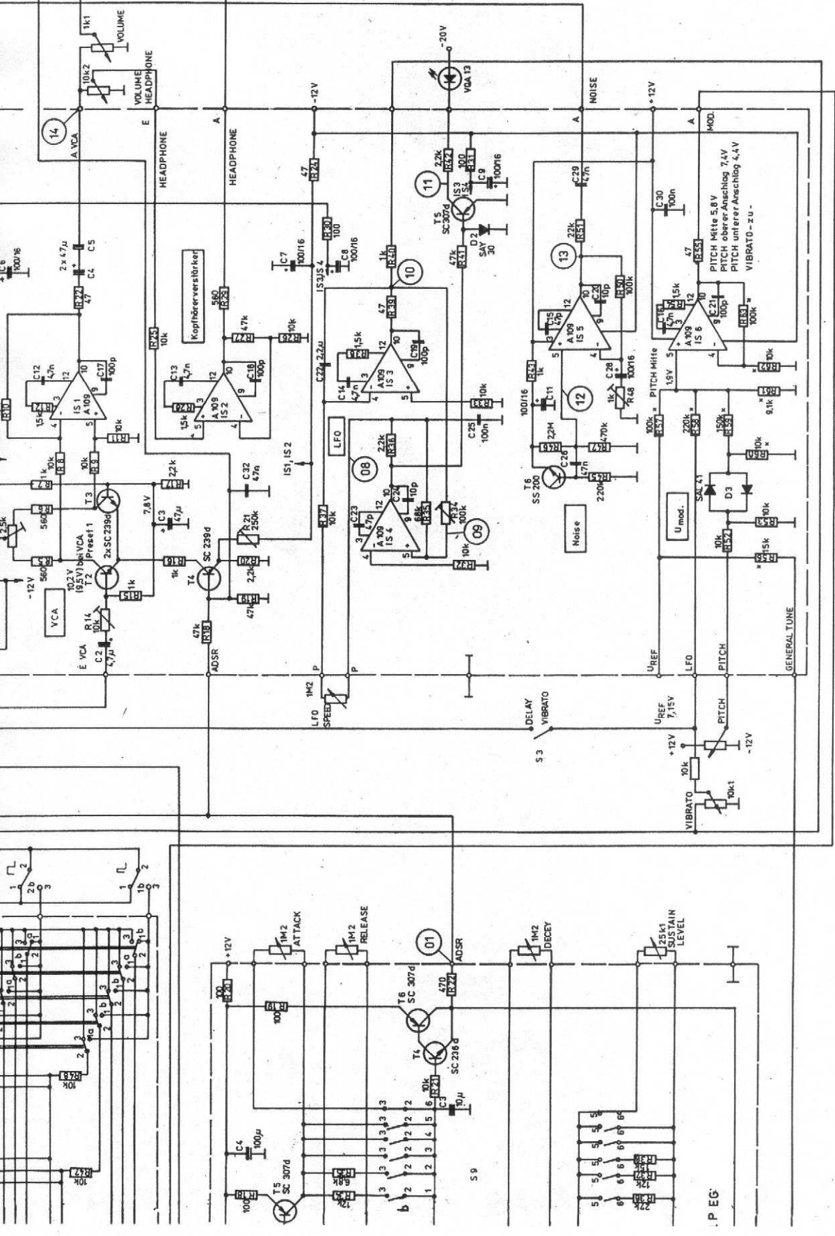
Gesamtstromlaufplan Synthesizer Общая коммутационная схема
